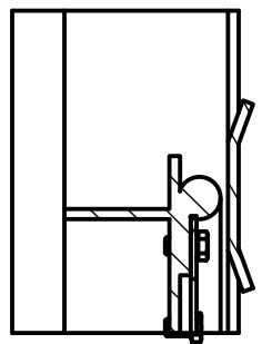
A-A ( 1 : 4 )
