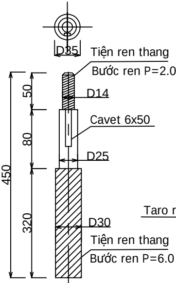
CHI TIẾT SỐ 2 DETAIL 2
