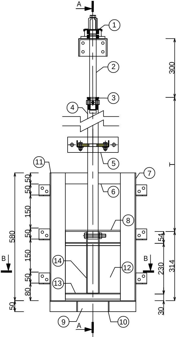
MẶT TRƯỚC ELEVATIONS VIEW
