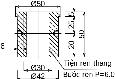
CHI TIẾT SỐ 3
