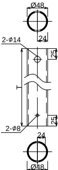
CHI TIẾT SỐ 4 DETAIL 4
