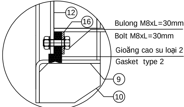
LIÊN KẾT GIOĂNG LOẠI 2 GASKET TYPE 2 LINK
