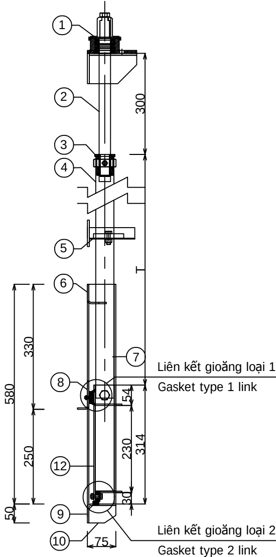
LIÊN KẾT GIOĂNG LOẠI 2 GASKET TYPE 2 LINK
